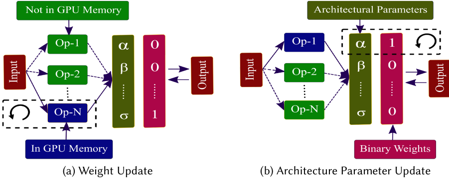
Fig. 7. ProxylessNAS [8].
